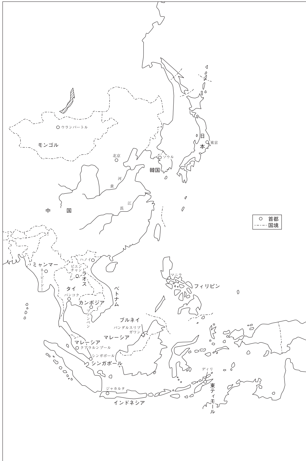
図-2 東アジア地域
