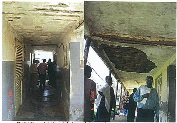
X線棟の中廊下(左)、病院中央の渡り廊下(右)ともにスラブの劣化が顕著である。
