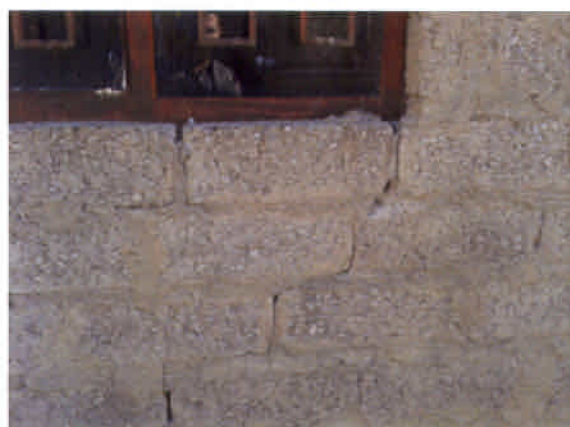
基礎工事がされていないため、壁に大きな亀裂が入り、倒壊の恐れがあり、生徒の身が危険である
