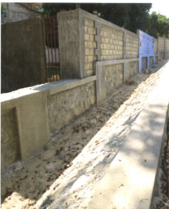
図2: 塀によりアクセス不可能な水源
