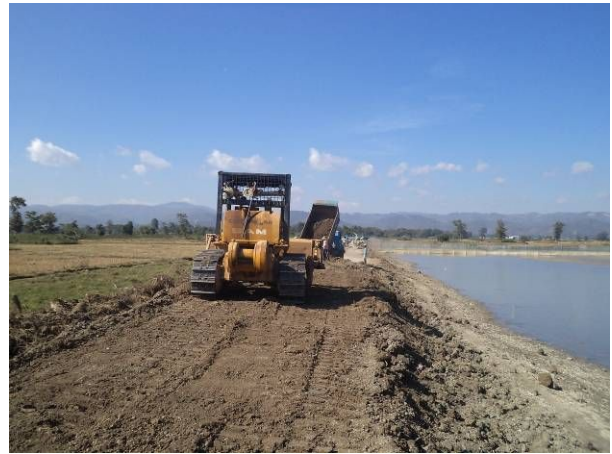
堤の工事(2011 年 12 月 17 日)
