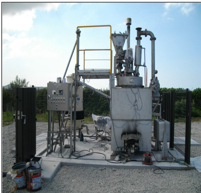
油化装置本体
