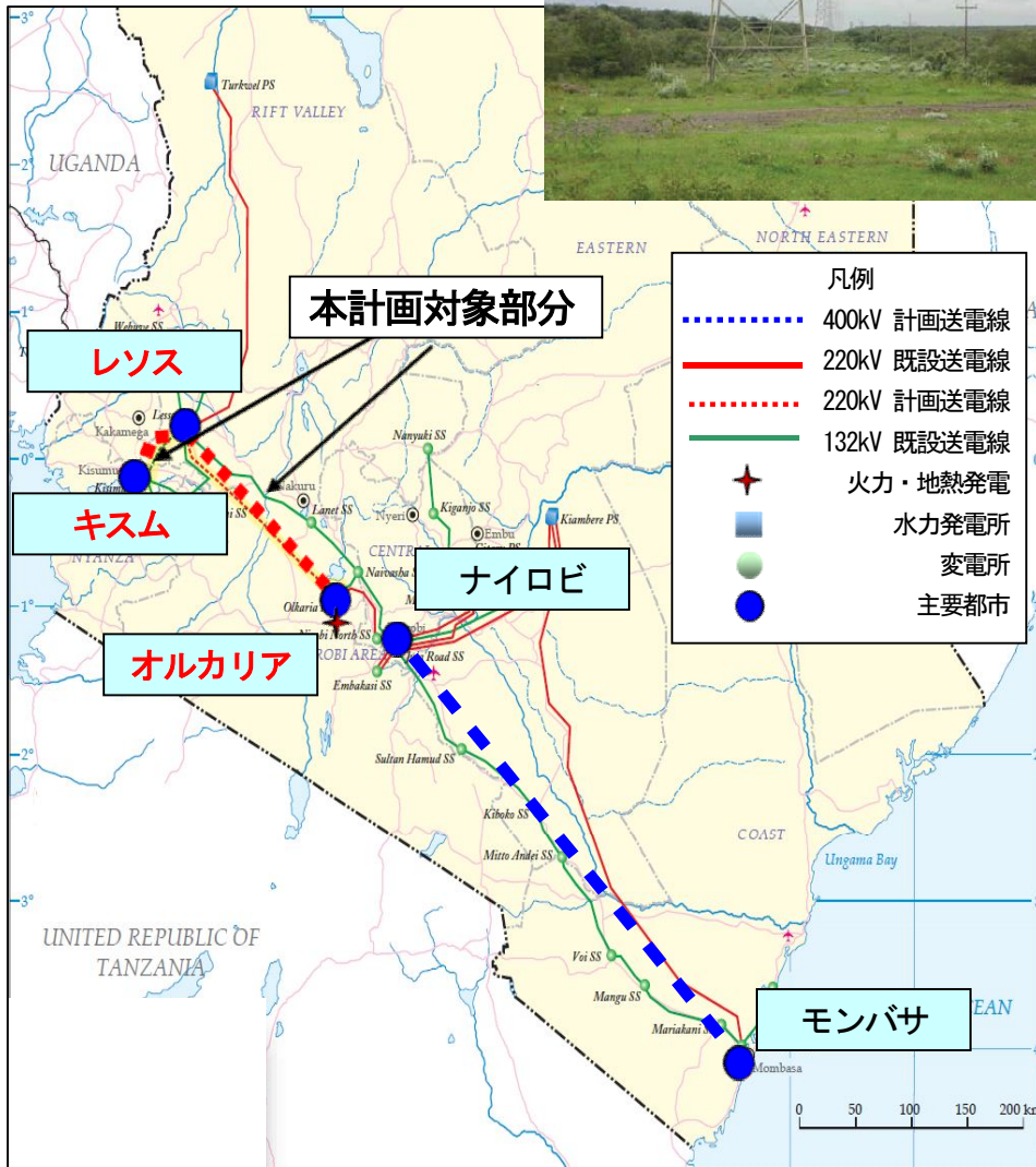
送電線建設位置図
