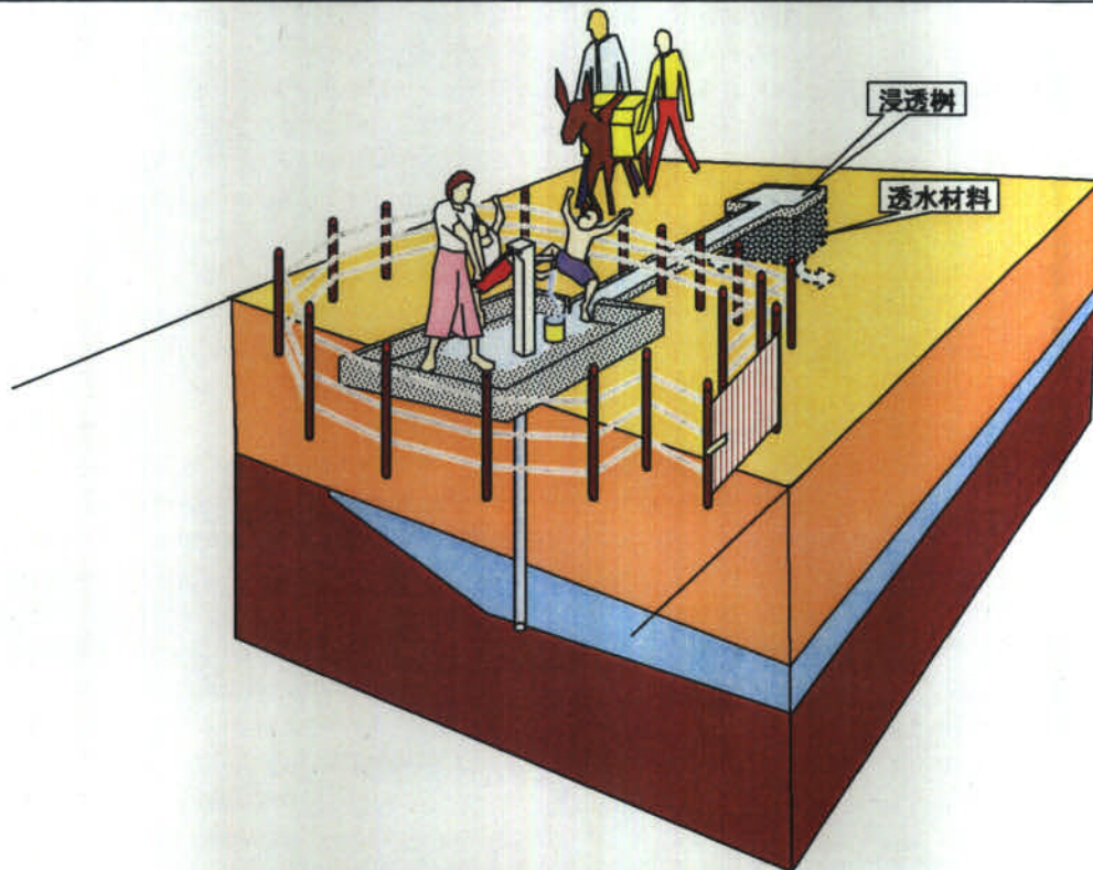
a) ハンドポンプ
