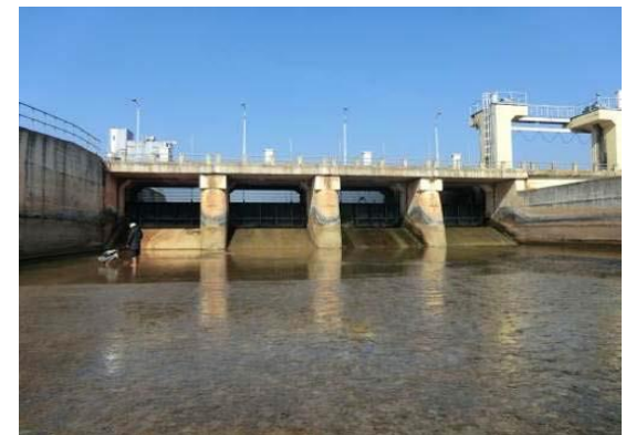
発電用取水ゲート全景
