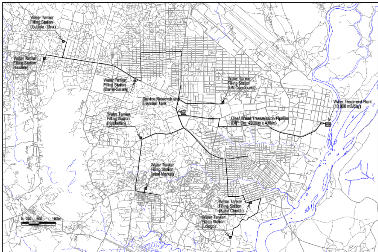
下:ジュバ市内主要施設位置図
