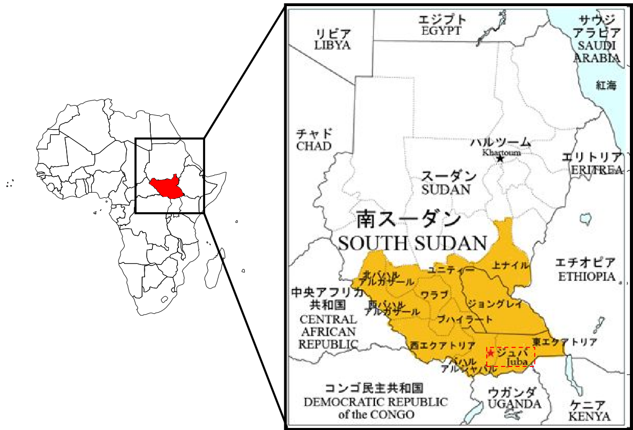
上:ジュバ位置図
