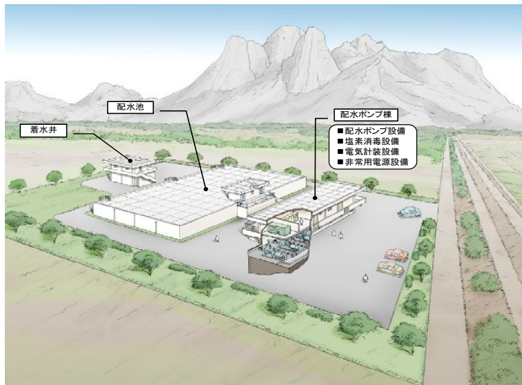
浄水場のイメージパース
